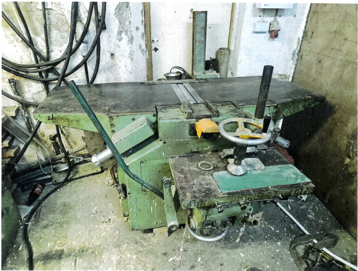
Fot. 1 Widok obrabiarki z przodu.
