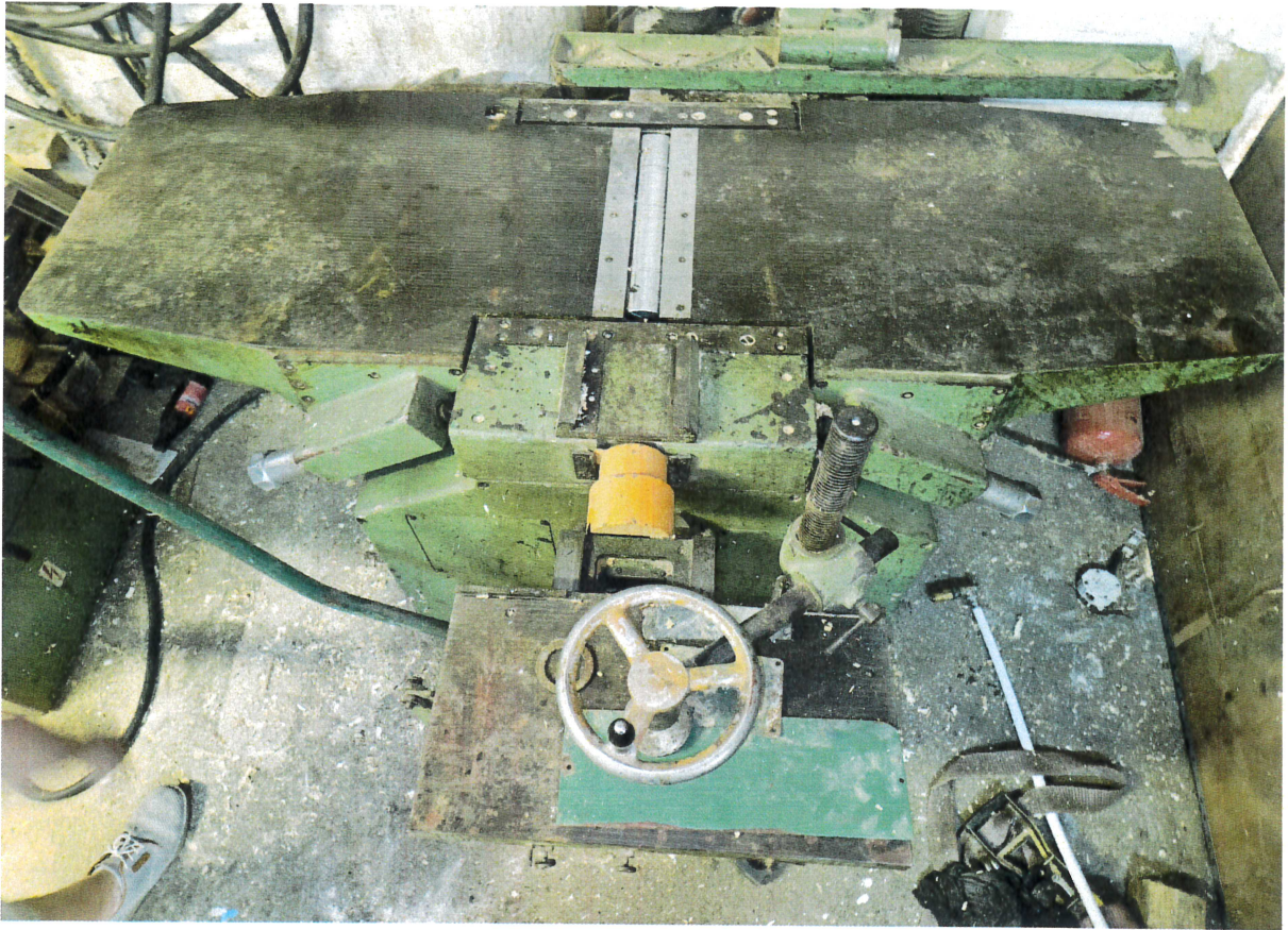
Fot. 4 Widok na stół roboczy maszyny.
